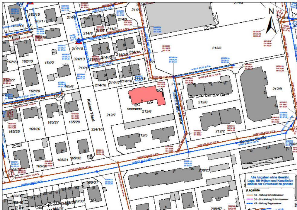
Abbildung 6: Schmutz- und Regenwasserkanäle sowie Anschlüsse
