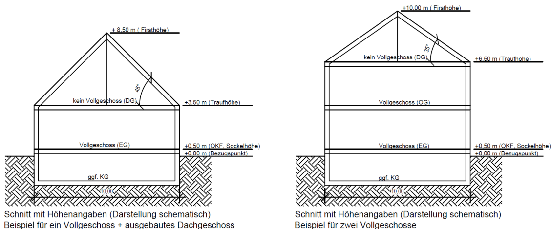
Abb. 5 Beispielhafte Gebäudeschnitte in ein- und zweigeschossiger Bauweise
